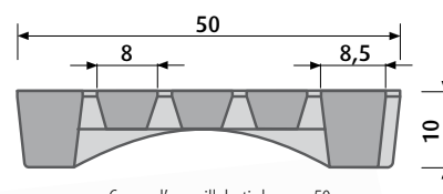
Coupe d'un caillebotis largeur 50 cm
