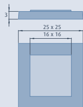
Semelle Tabernacle
