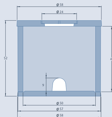
Citerneau rond
